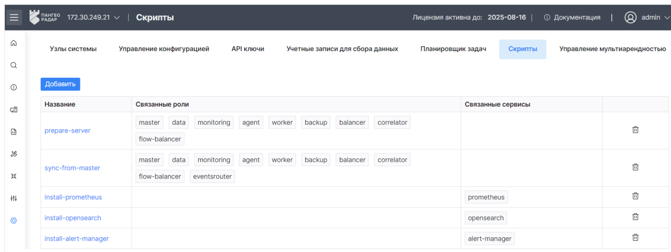
Рис. 128 – Раздел "Кластер". Вкладка "Скрипты"
