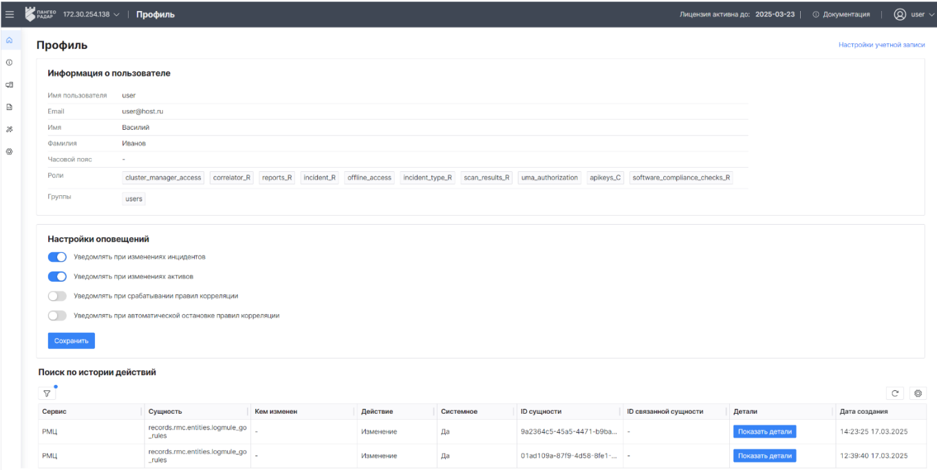
Рис. 150 – Раздел "Профиль"
