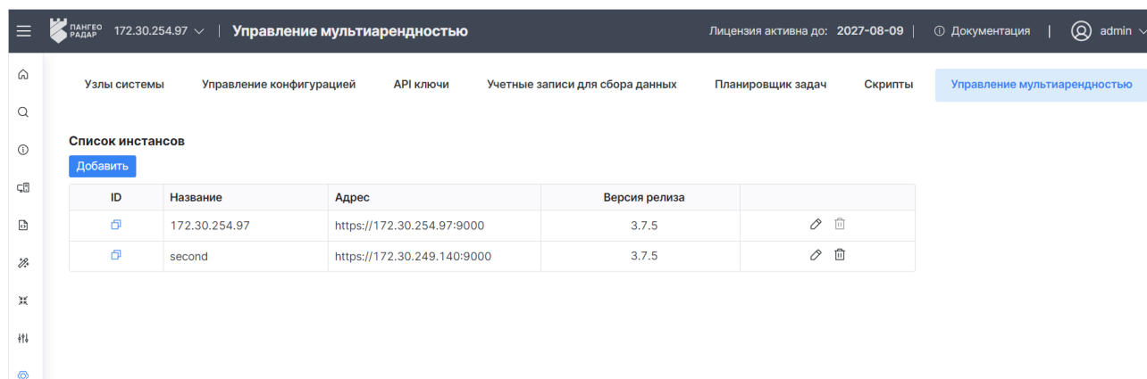
Рис. 133 – Раздел "Кластер". Вкладка "Управление мультиарендностью"
