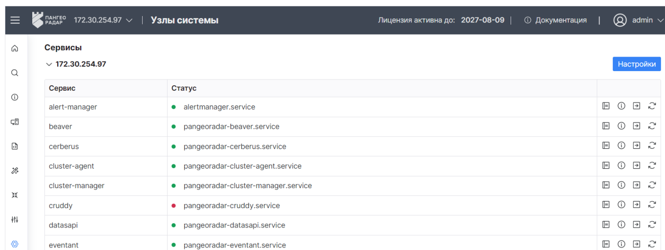
Рис. 113 – Блок "Сервисы"
