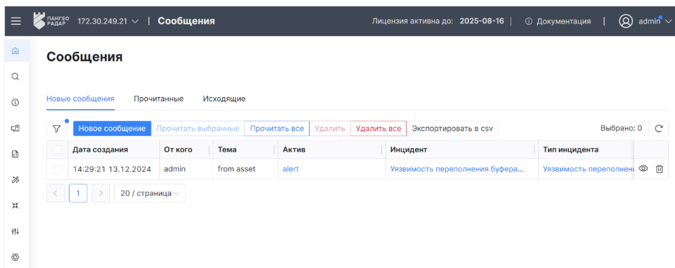
Рис. 147 – Раздел "Сообщения"
