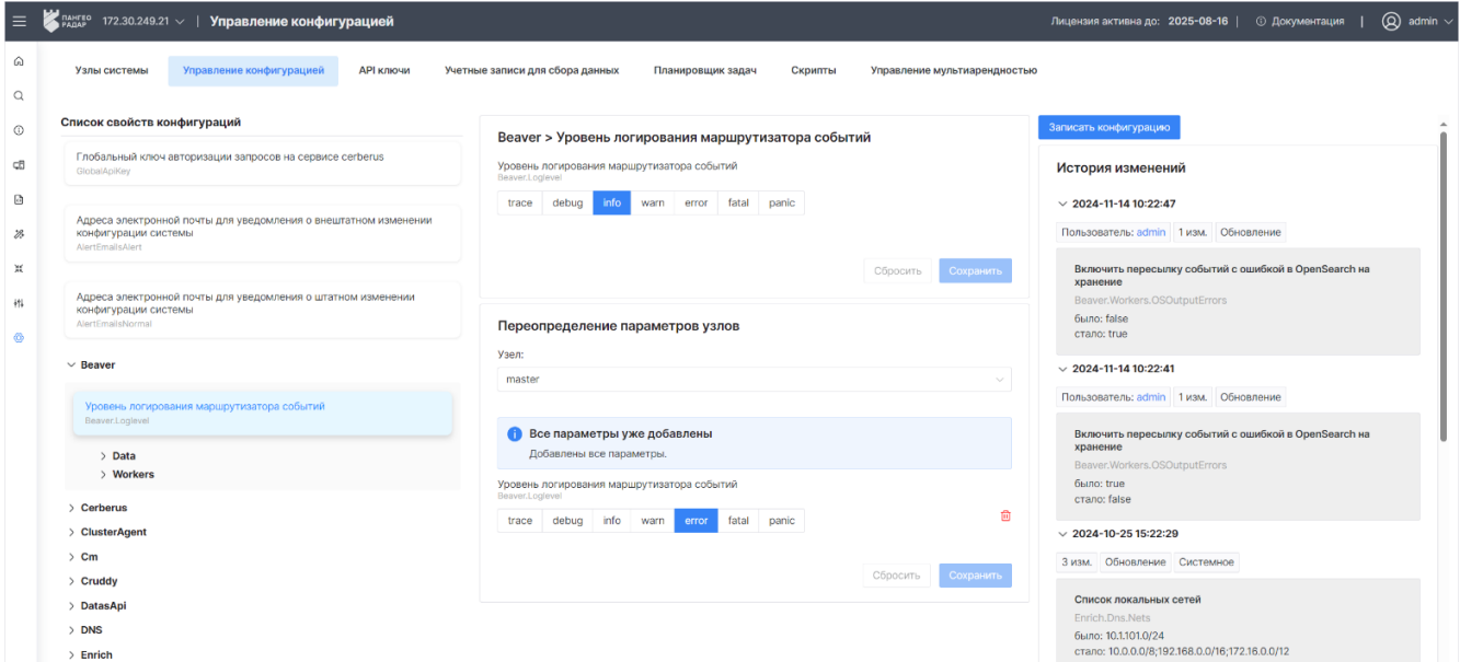
Рис. 116 – Раздел "Кластер". Вкладка "Управление конфигурацией"
