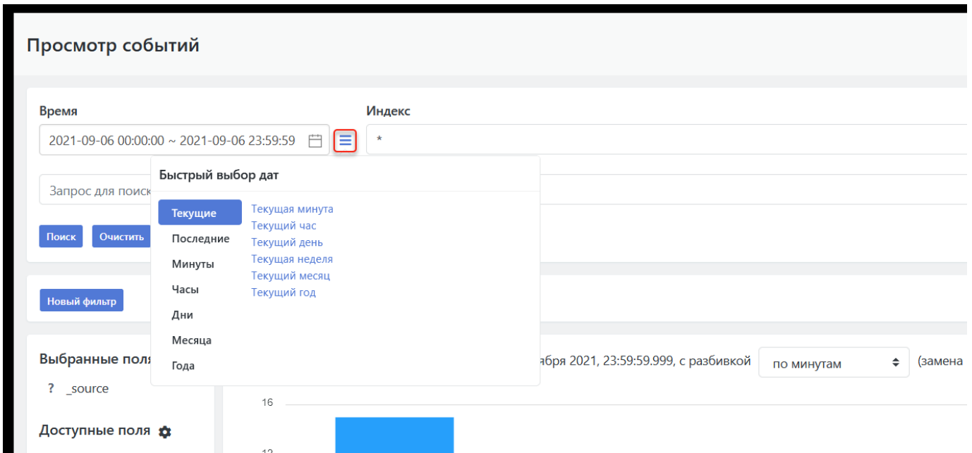
Рисунок 105 - Выбор предустановленного временного интервала для поиска событий
