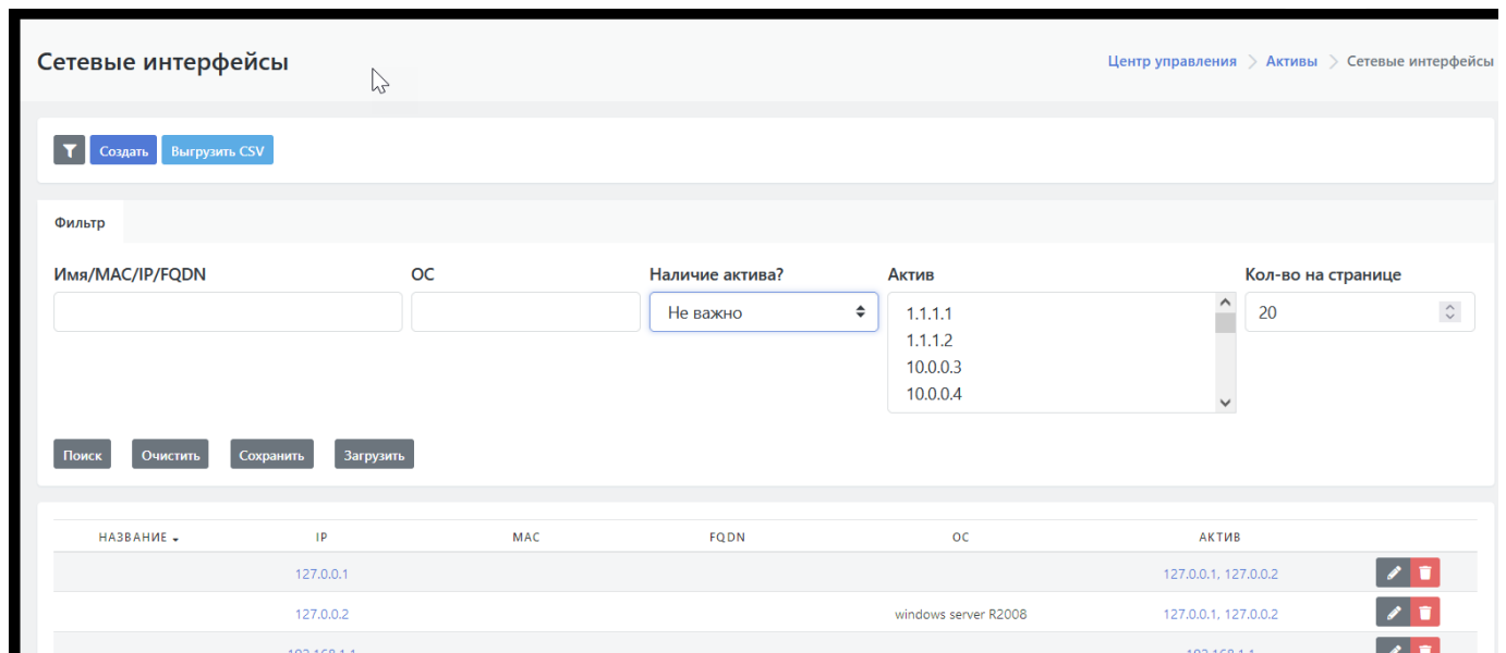
Рисунок 37 - Фильтр подраздела "Сетевые интерфейсы"
