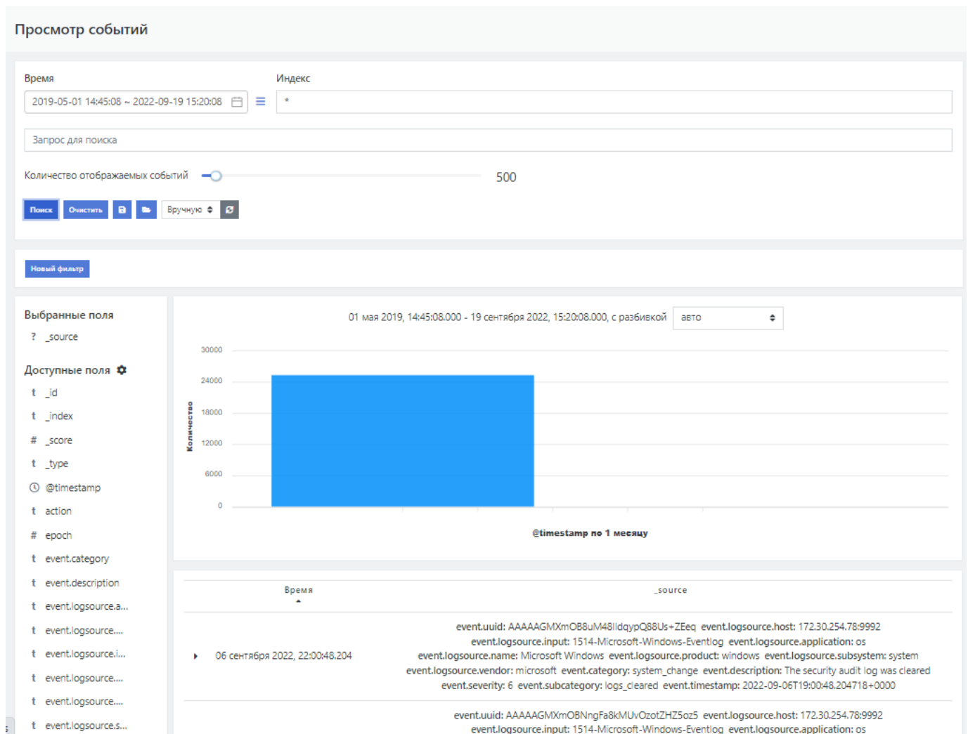
Рисунок 14 - Рабочая область подраздела «Просмотр событий»
