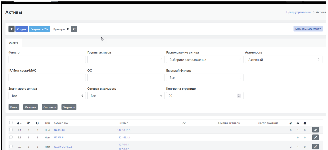
Рисунок 32 - Фильтры для списка активов
