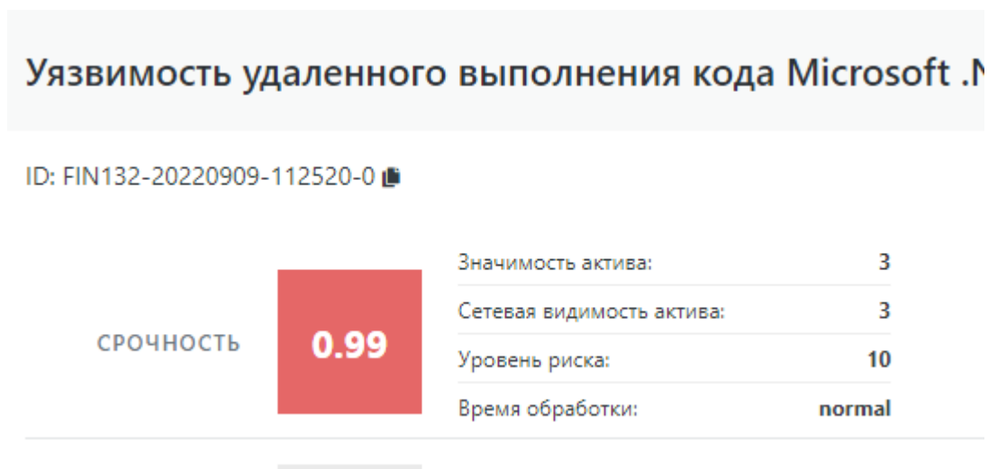
Рисунок 80 - Просмотр параметров, формирующих оценку срочности
